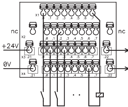
ricos COM 8I 8I/O
